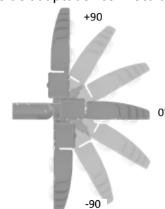
Inclinación Variable: De -90° a +90° Brazo de adaptador con rótula
