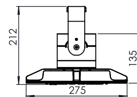
Dimensiones (mm):
